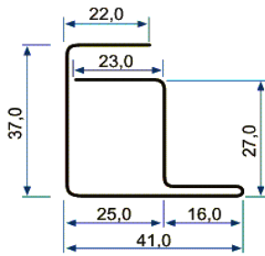
Perfil Leve 634 - Garra Contra Garra Linha 25 D
