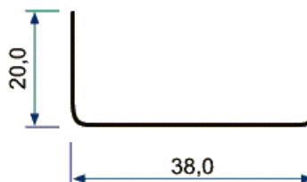
Perfil Leve 007 - Uzinho para Janela 3 mts
