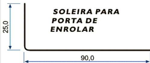
Perfil Leve 106 - Soleira para Porta de Enrolar
