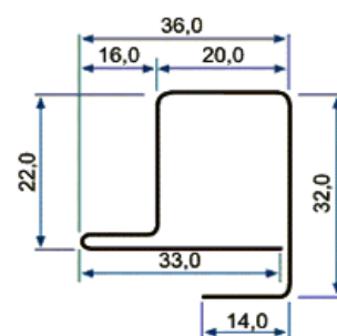
Perfil Leve 629 - Garra Contra Garra Linha 20 B
