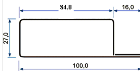
Perfil Leve 105 - Cant. Cadeira para Porta
