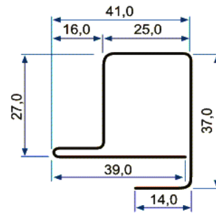
Perfil Leve 633 - Garra Contra Garra Linha 25 E
