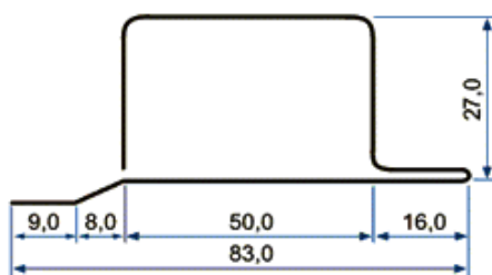
Perfil Leve 626 - T Porta Vedação Linha 50
