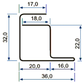
Perfil Leve 630 - Garra Contra Garra Linha 20 C
